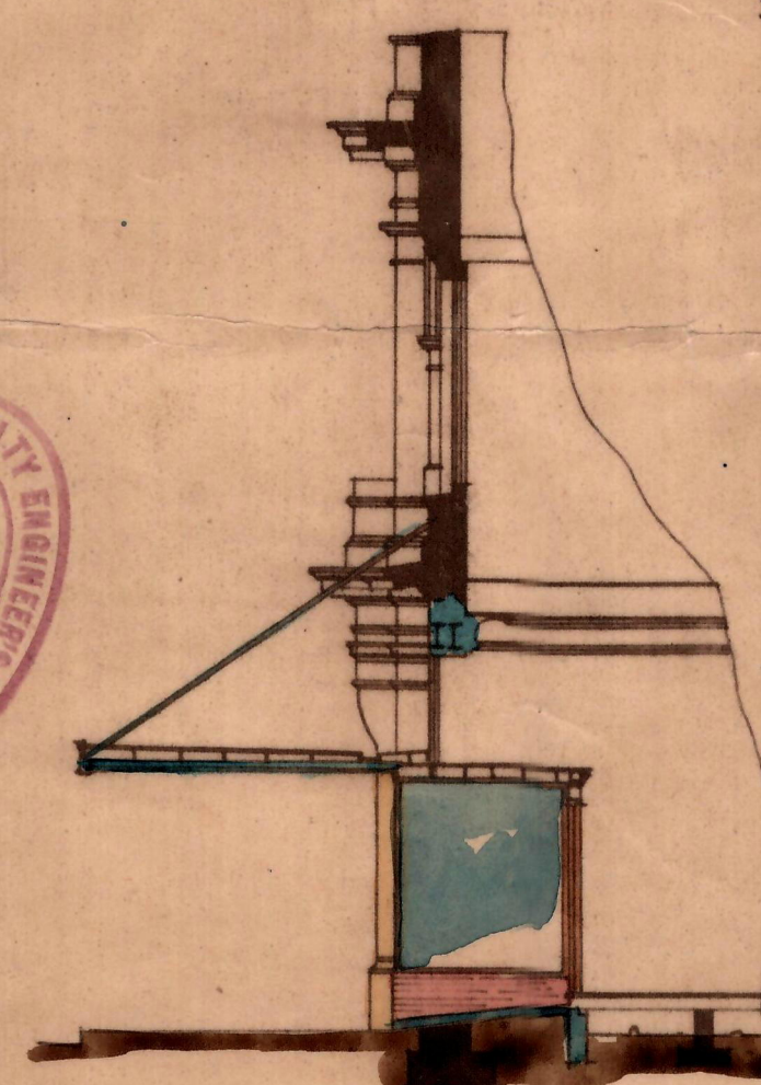
SECTION A-B
