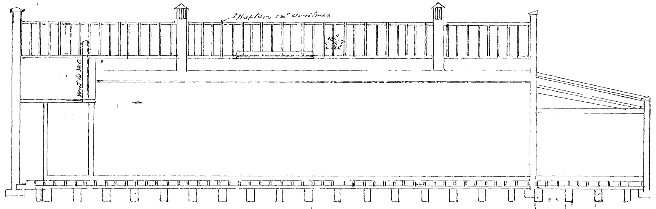
— Longitudinal Section —
